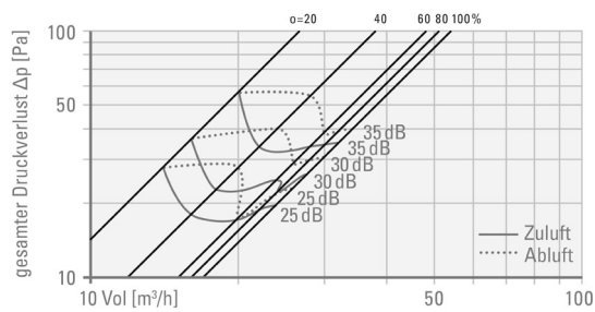
VAZAM100 mit Luftregulierung
