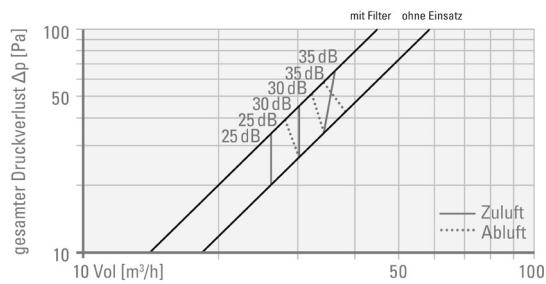
VAZAM 100 mit Staubpartikelfilter/ohne Staubpartikelfilter
