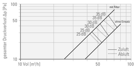
VAZUM 100 mit Staubpartikelfilter/ohne Staubpartikelfilter
