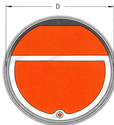
Vue en coupe KRSM, variante montage dans un tube
