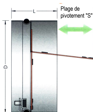
Vue en coupe KRSM, variante montage dans un tube
