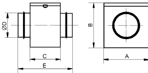
Luftfilterboxen
