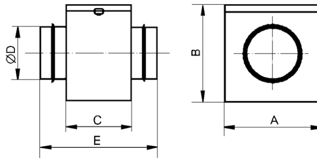
Caisson filtre à air LFB
